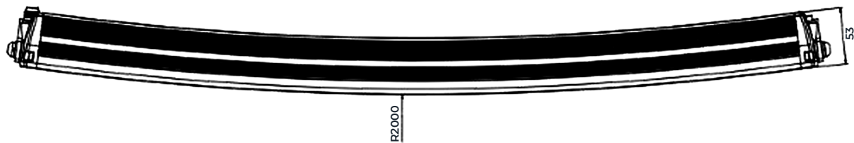
Figur 2 Ovenfra — bueradius R2000, dybde 53 mm
