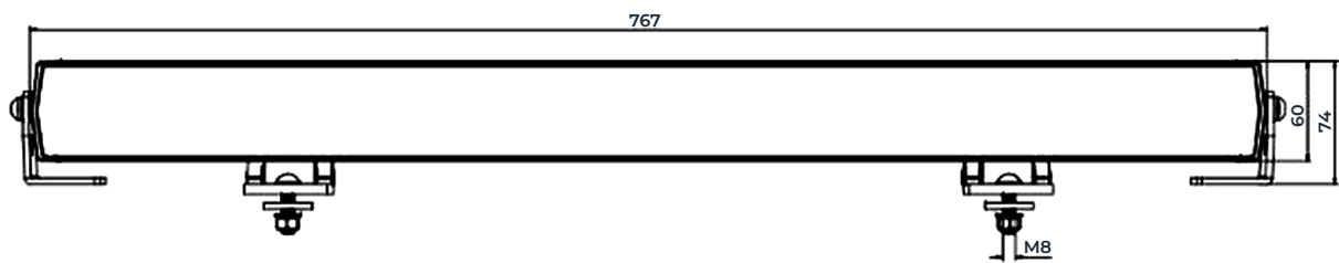
Figur 1 Forfra — alle mål i mm
