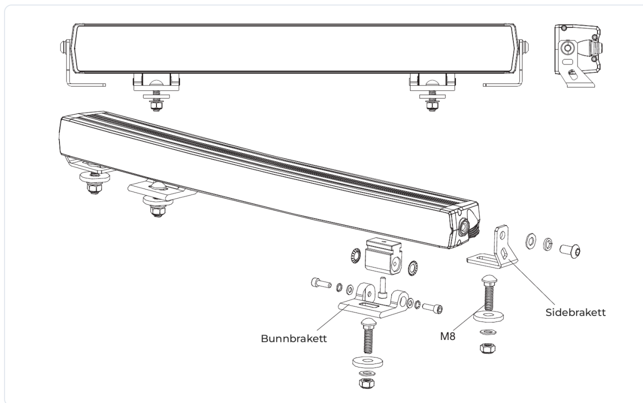
Figur 4 Montering med bunnbrakett eller sidebrakett, festebolt M8
